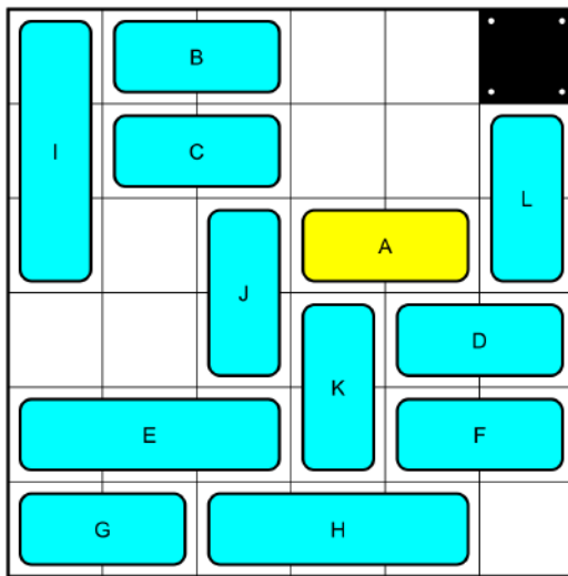
24 Moves_No48537.png
