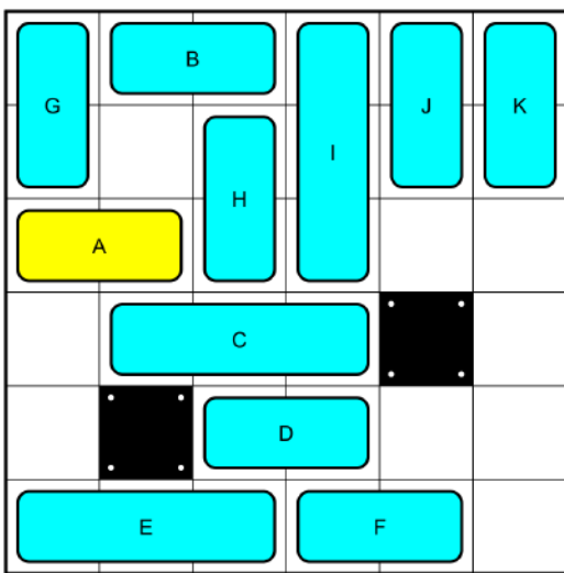
29 Moves_No10649.png
