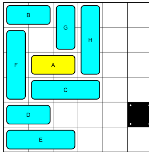
24 Moves_No49910.png
