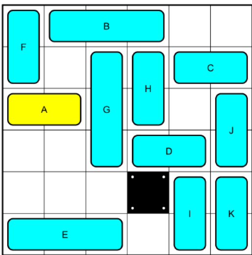
17 Moves_No358805.png
