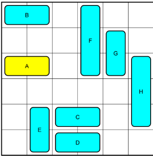
14 Moves_No842952.png
