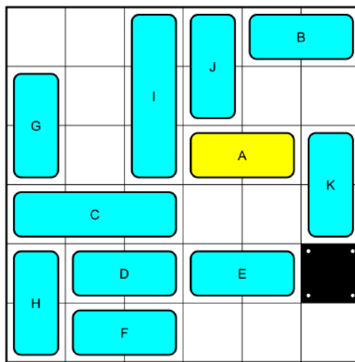
13 Moves_No970761.png
