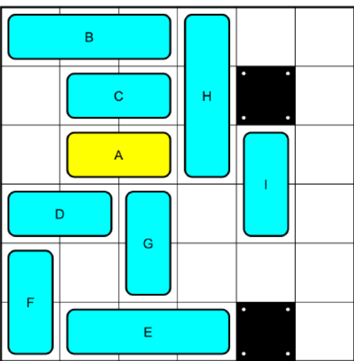
11 Moves_No1431888.png
