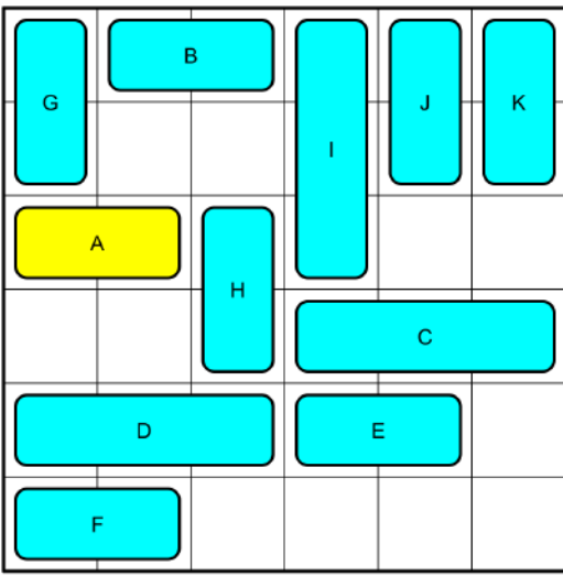
30 Moves_No7341.png
