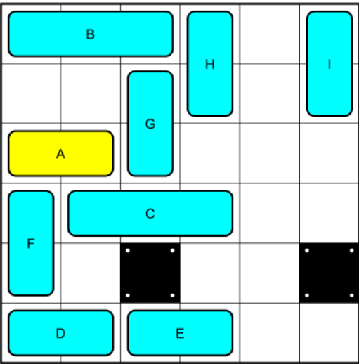
13 Moves_No879743.png
