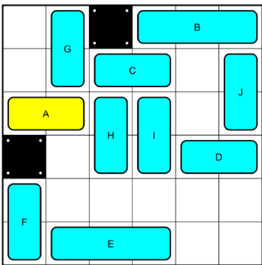
12 Moves_No1160532.png
