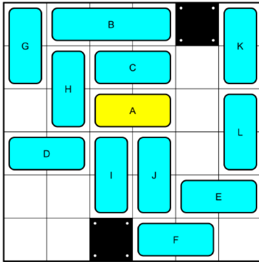
16 Moves_No529993.png
