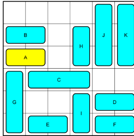
13 Moves_No906023.png
