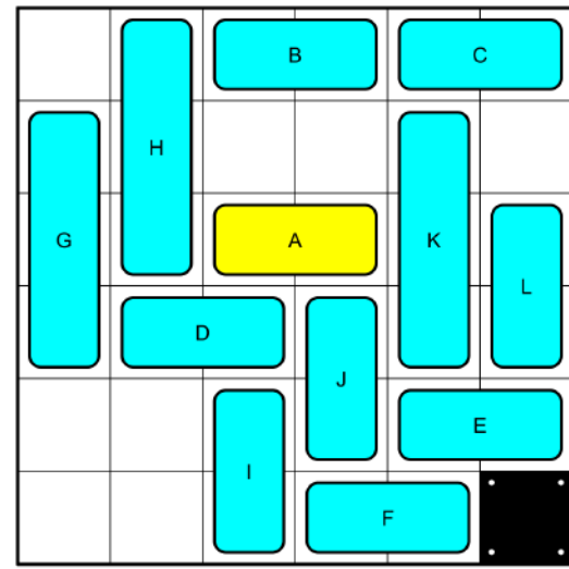
30 Moves_No7446.png
