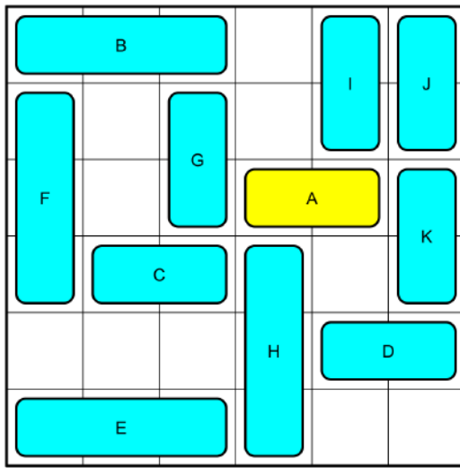
32 Moves_No4126.png
