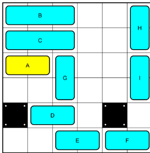
13 Moves_No958372.png
