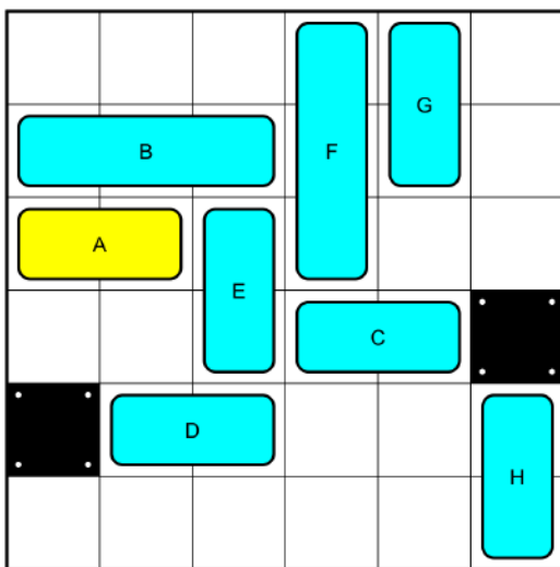
10 Moves_No1845986.png
