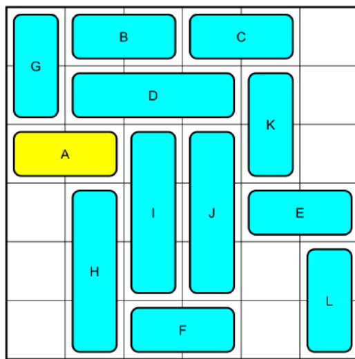
17 Moves_No363951.png
