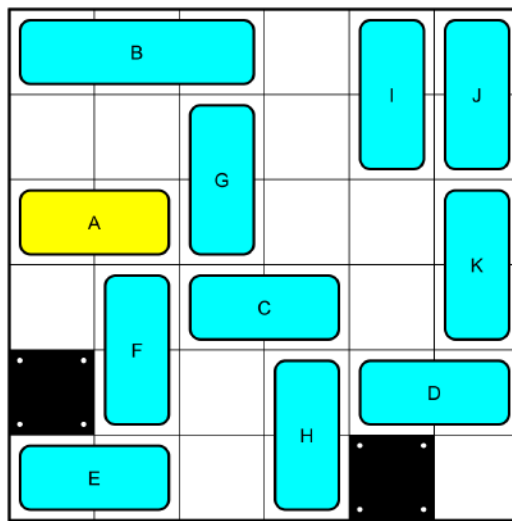
22 Moves_No82383.png
