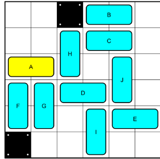
30 Moves_No9026.png
