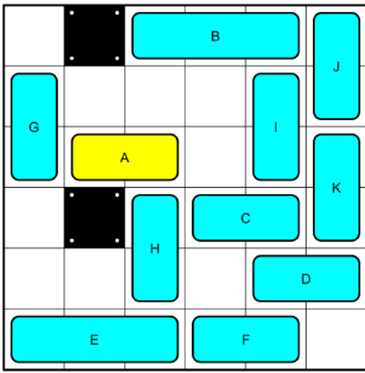
15 Moves_No597980.png
