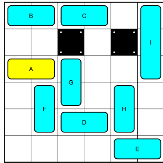
15 Moves_No545705.png
