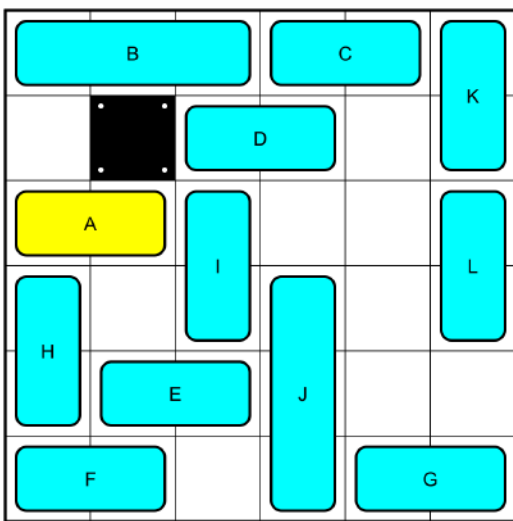
27 Moves_No19731.png
