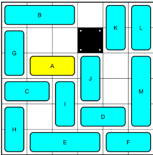
20 Moves_No180847.png
