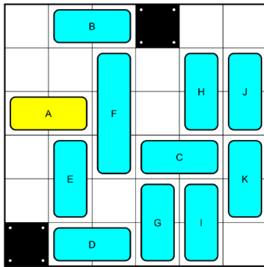
15 Moves_No556488.png
