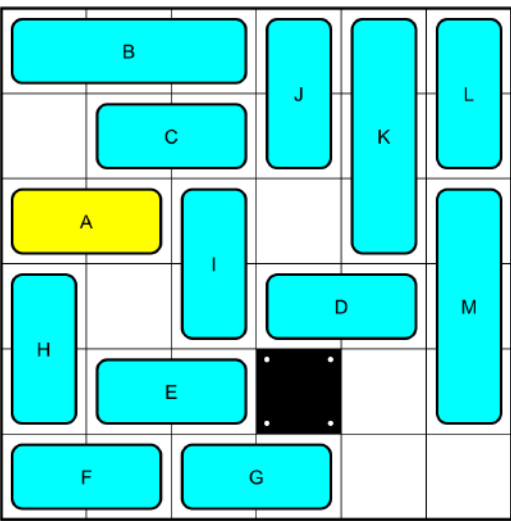
31 Moves_No5921.png
