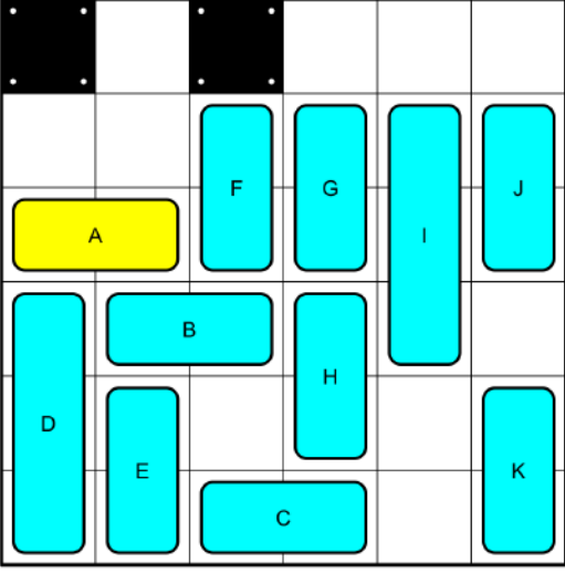
25 Moves_No30394.png
