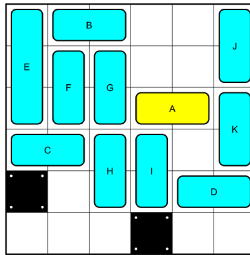
32 Moves_No4444.png
