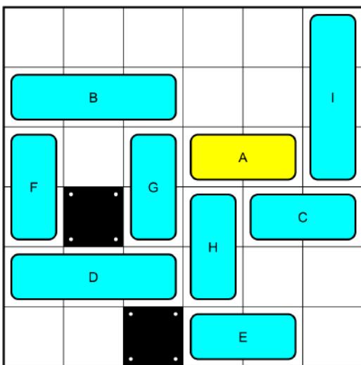
26 Moves_No29121.png
