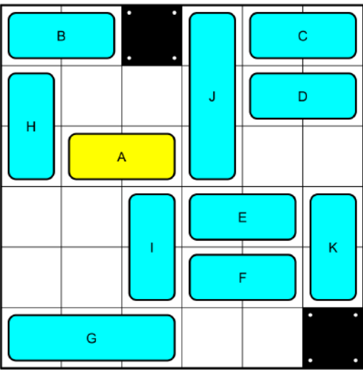
21 Moves_No111117.png
