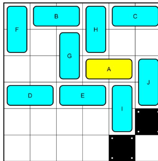
13 Moves_No855306.png
