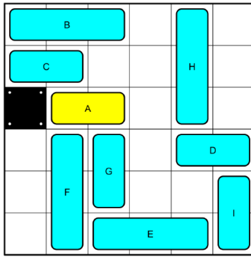
15 Moves_No603080.png
