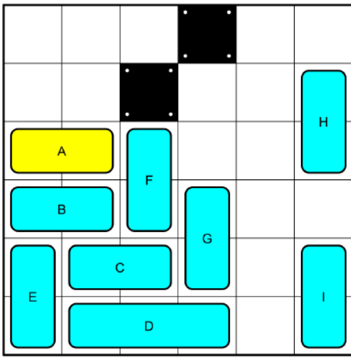
16 Moves_No453170.png
