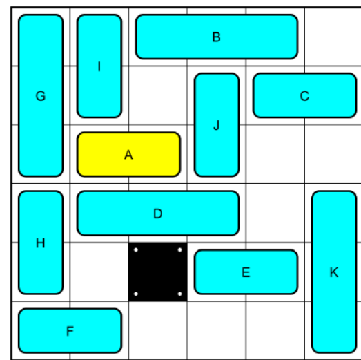
24 Moves_No43413.png
