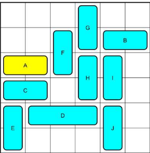
31 Moves_No6733.png
