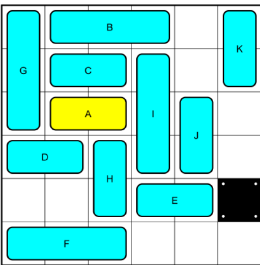
27 Moves_No18567.png
